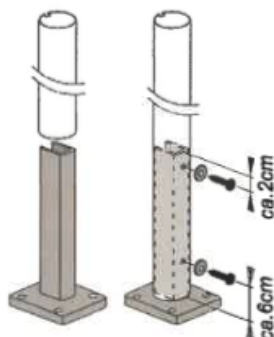
Aufsteck-Dübelkonsolen Ø60
